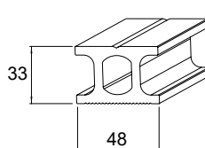
Опорная лага (ПВХ)
